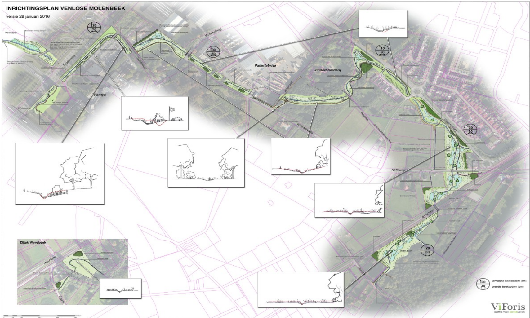
Inrichtingsplan Venlose Molenbeek (2,4 km)
